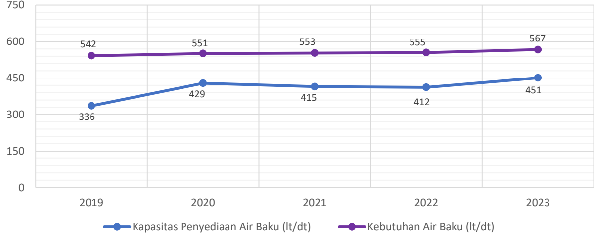
Sumber : Perumdam Tirta Taman, 2024 dan Analisis Bapelitbang, 2024 Gambar 2. 22 Kuantitas Penyediaan Air Baku
