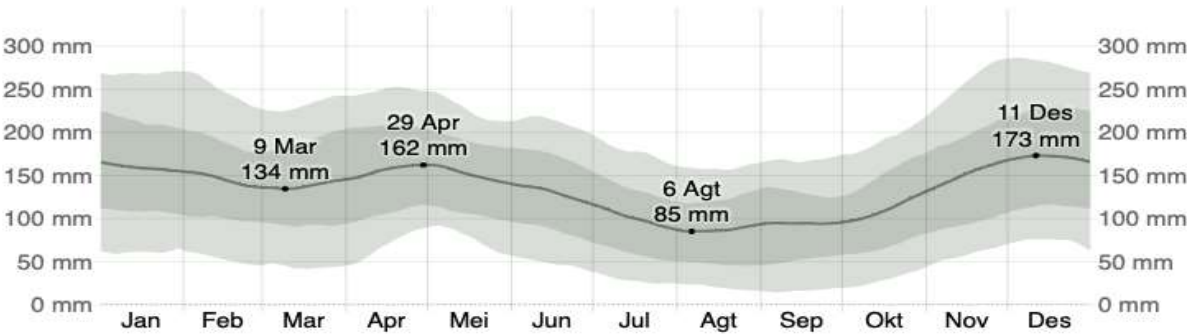
Gambar 2. 6 Rata-rata Curah Hujan Bulanan Kota Bontang
