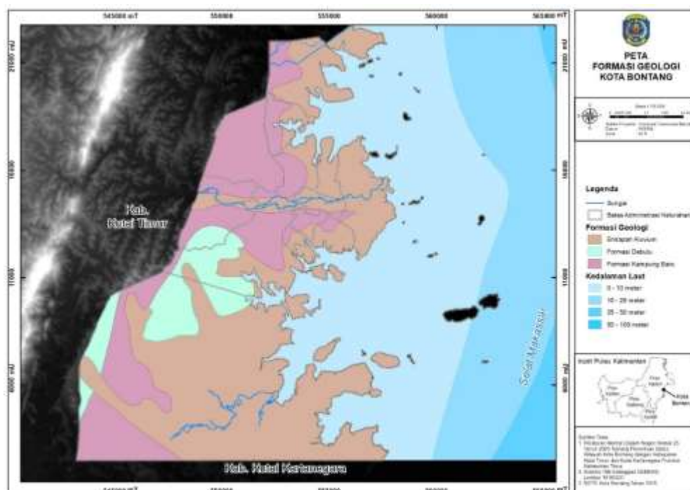
Gambar 2. 4 Peta Formasi Geologi Kota Bontang
